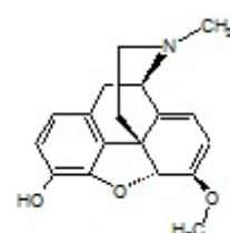
Oripavine
