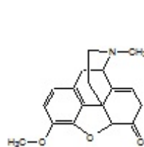
Neopinone
