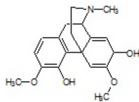
Salutaridinol
